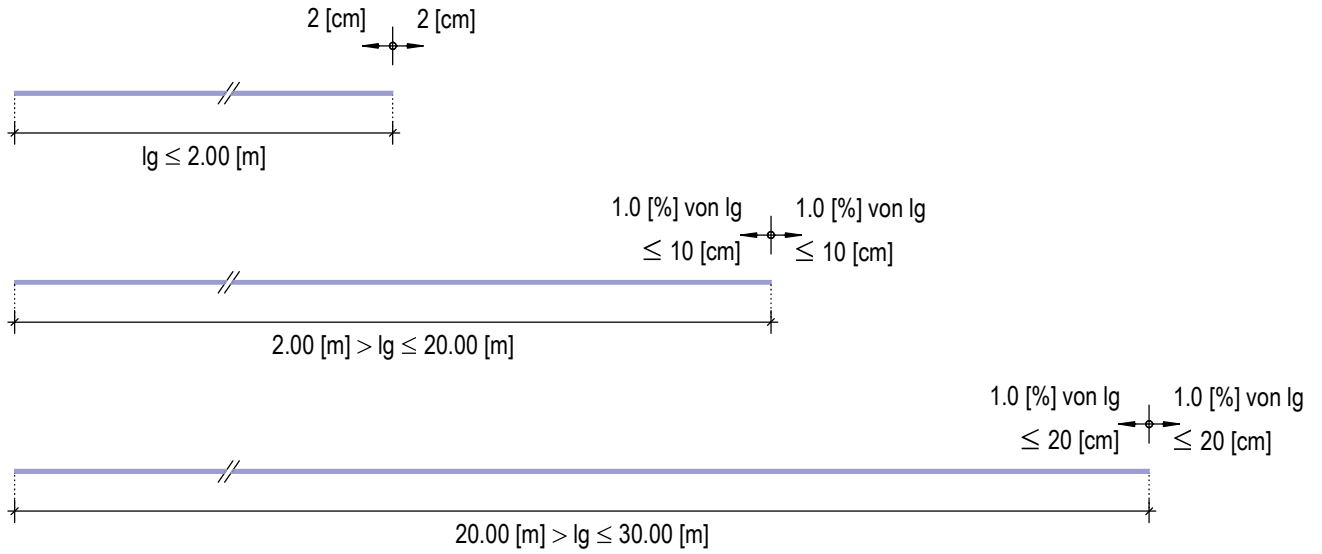
Bild 1.56 Toleranzen für geschnittene gerade Bewehrungen
