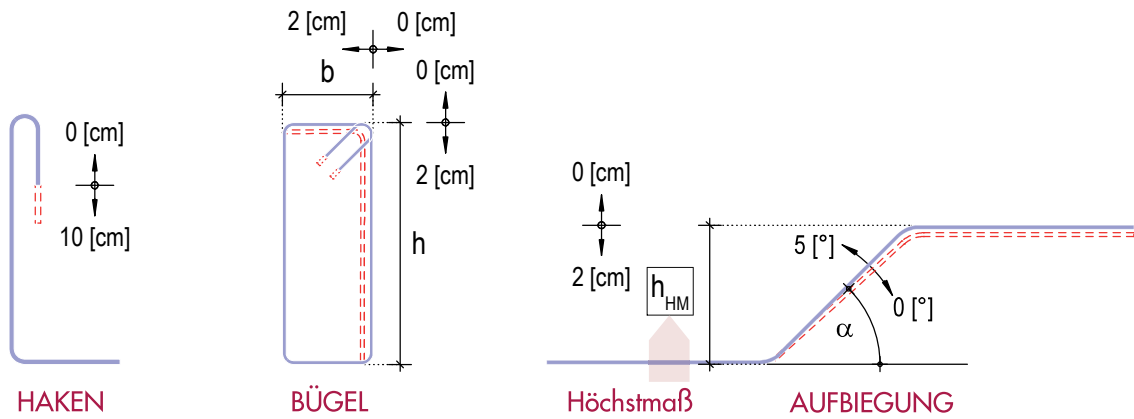
Bild 1.57 Toleranzen für gebogene Bewehrungen
